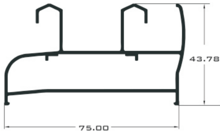
4601 CERCO PERIMETRAL
